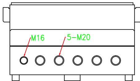
( 정면도 )
