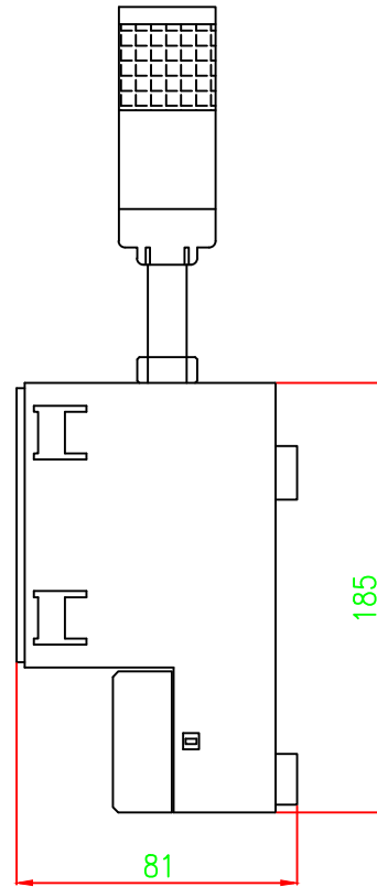
( 측면도 )
