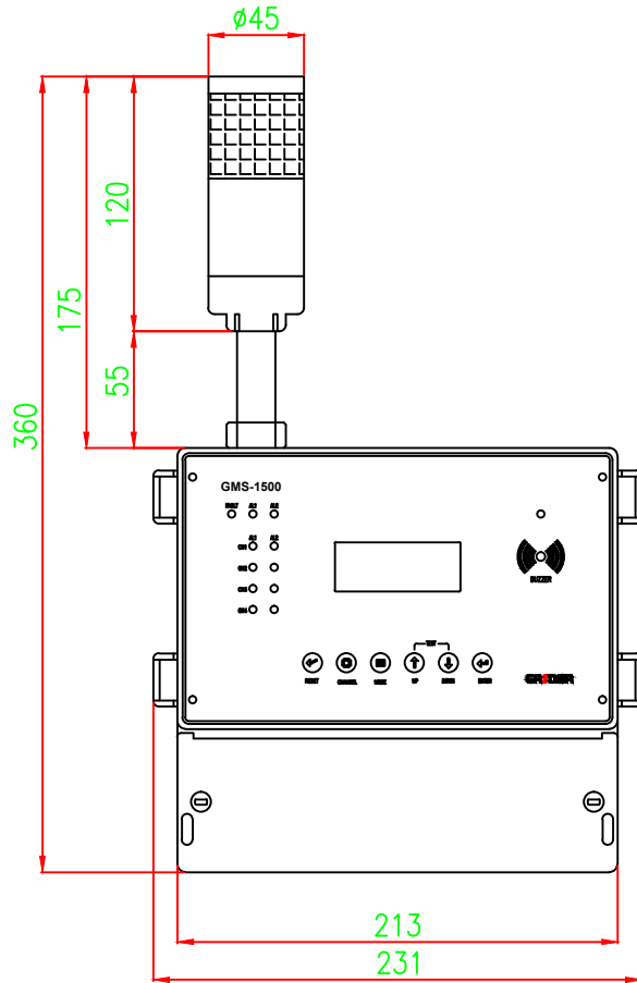
( 평면도 )
